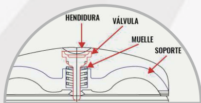
VÁLVULA DE SEGURIDAD
